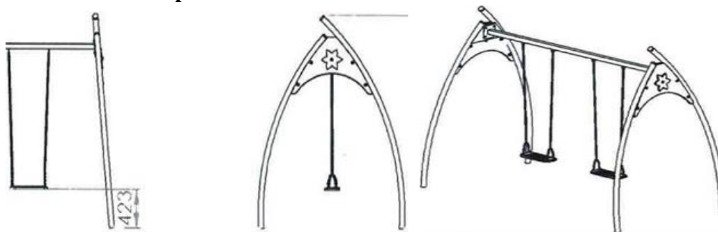
Dimensiunile echipamentului CL - 204
